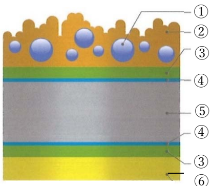
塗膜構成イメージ図
