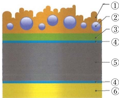
塗膜構成イメージ図
